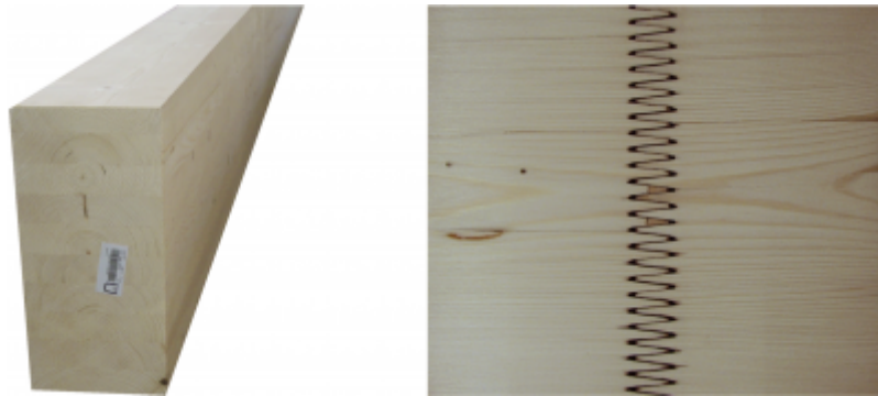
Abb. 3: Brettschichtholz; Keilzinkung einer BSH-Lamelle
