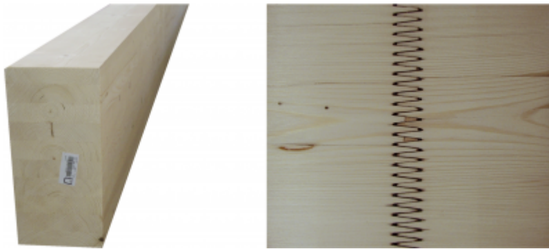
Abb. 3: Brettschichtholz; Keilzinkung einer BSH-Lamelle
